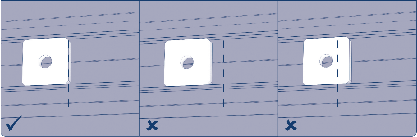
Рис. 7. Позиционирование закладной шайбы с левой стороны герметизатора
